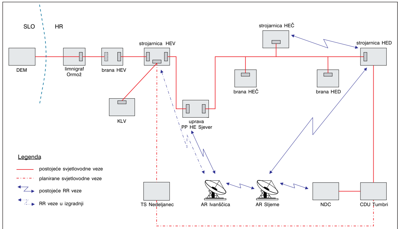
Slika 2. Shematski prikaz telekomunikacijskih sustava
