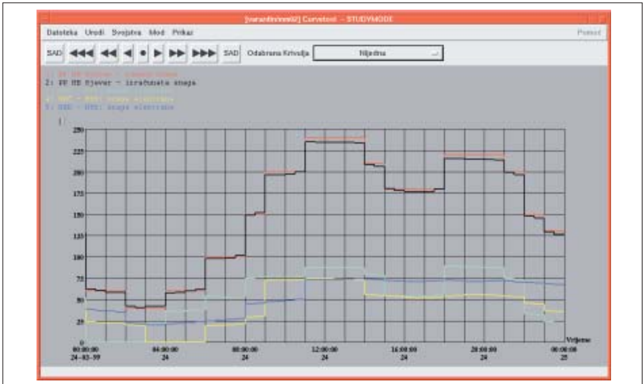
Slika 5. Prikaz rezultata proračuna programa HYS
