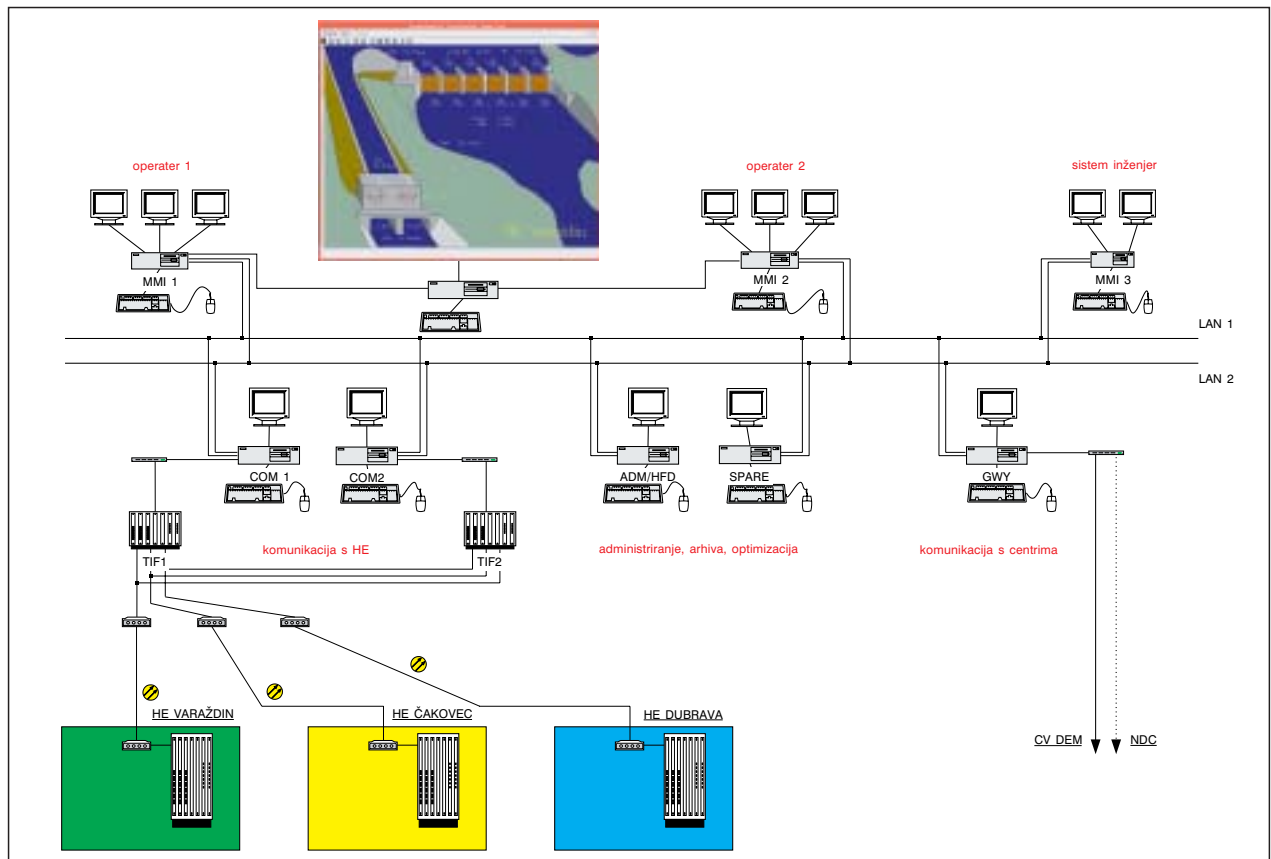
Slika 1. Shematski prikaz računarske opreme Komande lanca Varaždin
