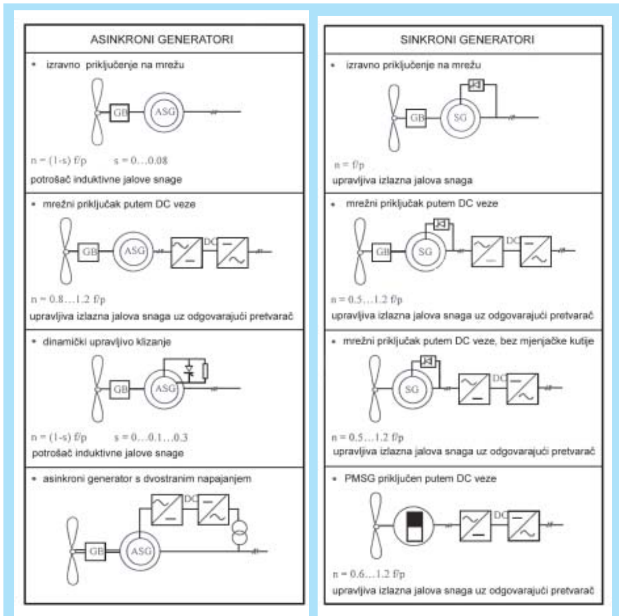
Slika 3. Vrsta priključenja vjetroelektrane na mrežu
