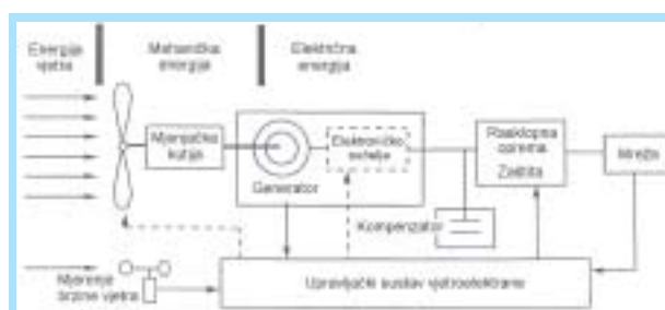
Slika 1. Općenita shema djelovanja vjetroelektrane
