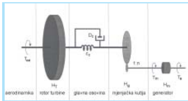
Slika 14. Dvomaseni evivalent pogonskog sustava
