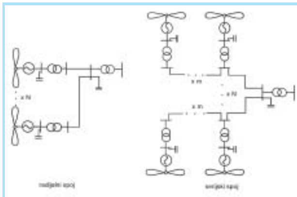
Slika 7. Osnovne konfiguracije priključenja agregata unutar vjetroelektrane
