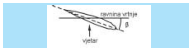
Slika 9. Kut zakreta elisa propelera \beta
