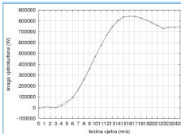
Slika 15. Ovisnost snage vjetroturbine o brzini vjetra
