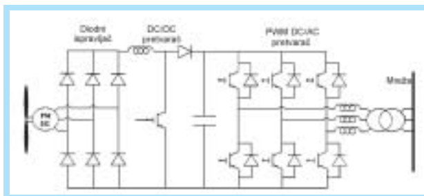
Slika 5. Vjetroelektrana u izvedbi s promjenjivom brzinom vrtnje koja koristi sinkroni generator s permanentnim magnetima bez mjenjačke kutije
