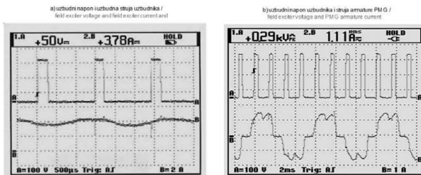
Slika 10 — Stacionarno opterećenje generatora, mjereni oblici Figure 10 — Generator steady loading, measured waveforms
